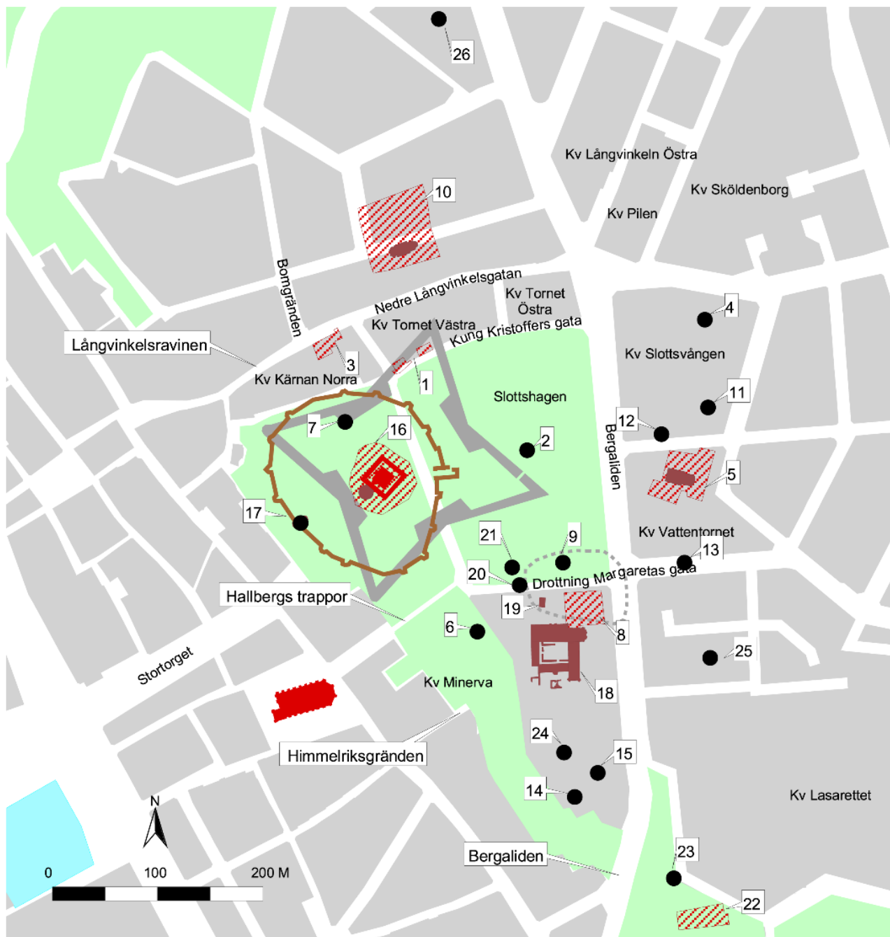
Fig. 5. Bebyggelselämningar på landborgen. Befintliga medeltida byggnader är rödskräfferade medan arkeologiskt dokumenterade och icke kvarstående byggnader i murverk på landborgen har brunskräfferats. Den medeltida borgansläggningen (med ringmur och borgtorn) samt kastellet, anlagt 1658-1678, är markerade. Utbredningen av sänkan norr om dominikankonventet markeras av grå streckad linje. Referenser till de arkeologiska observationerna finns i texten. Skala 1:6 000.
